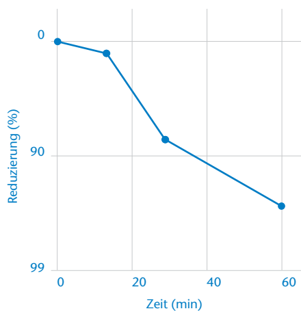
MS2-Bakteriophagen-Virus
